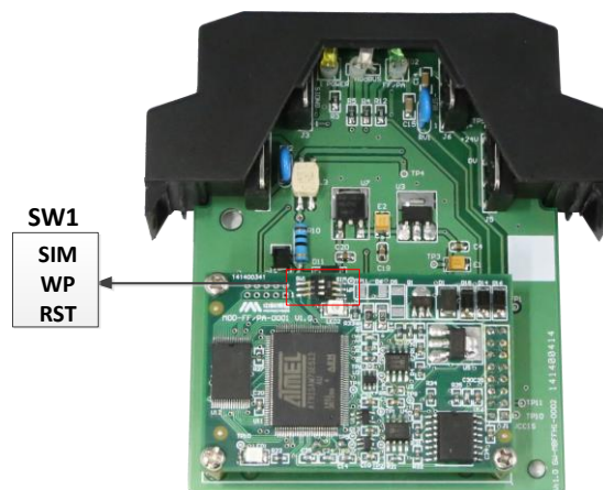
图 2.2 G0313 Modbus 转 FF 网关拨码开关
