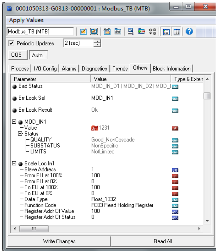
图 4.4 Modbus 寄存器配置
