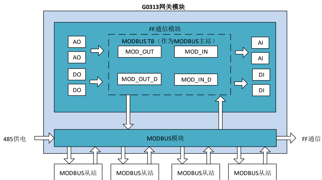
图 3.2 Modbus 转 FF 网关模块原理框图
