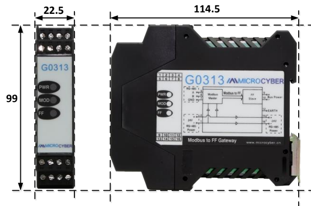
图 1.2 网关设备外型尺寸（单位：mm）
