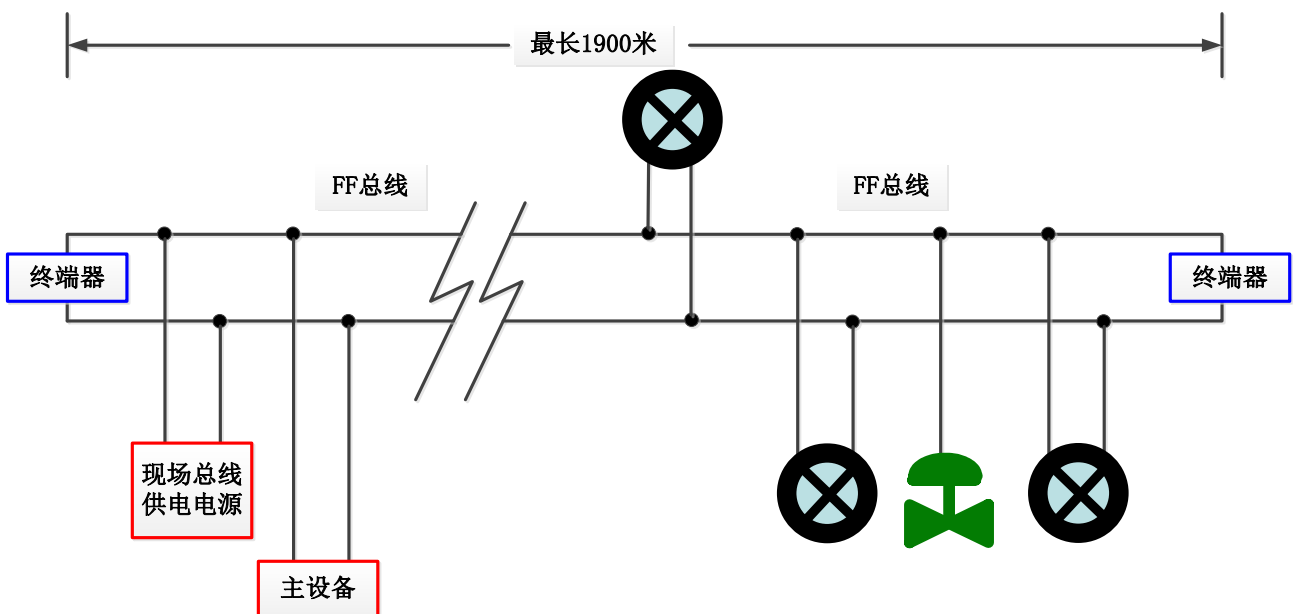
图 4.2 FF 总线连接
