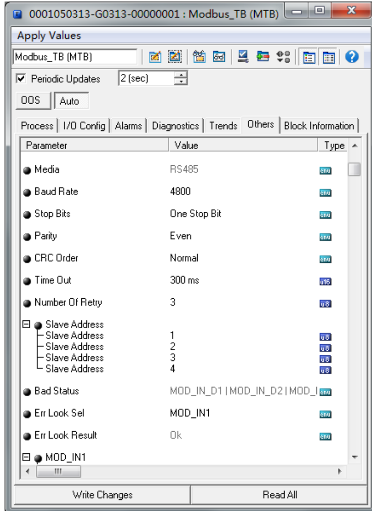
图 4.3 Modbus 通信参数配置
