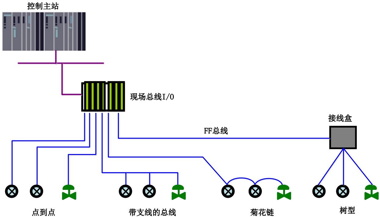
图 4.1 FF 网络拓扑
