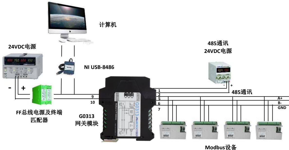
图 3.1 Modbus 转 FF 网关模块系统连接
